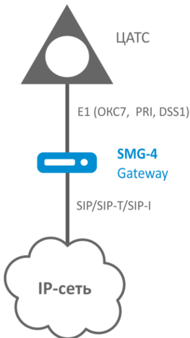
Рисунок 1 - Подключение к IP-сети через транковый шлюз SMG-4
