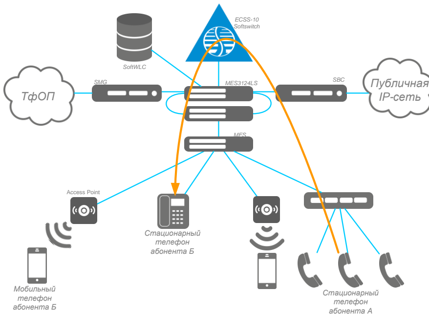
Рисунок 2 – Схема прохождения вызова абонента А абоненту Б
