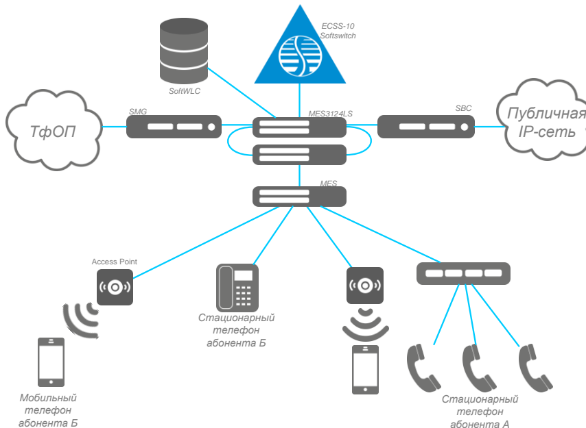
Рисунок 1 – Схема использования SIP-клиента с ECSS-10 Softswitch
