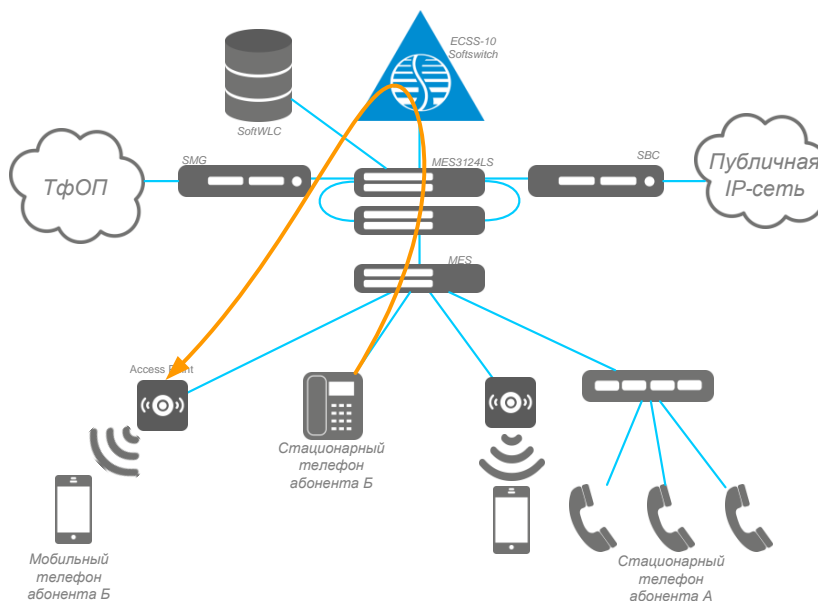
Рисунок 3 – Схема прохождения вызова абонента А абоненту Б
