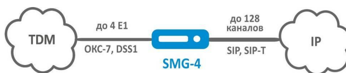
Рисунок 1 – Сопряжение сигнализаций и медиапоточков TDM- и VoIP-сетей с использованием SMG-4
