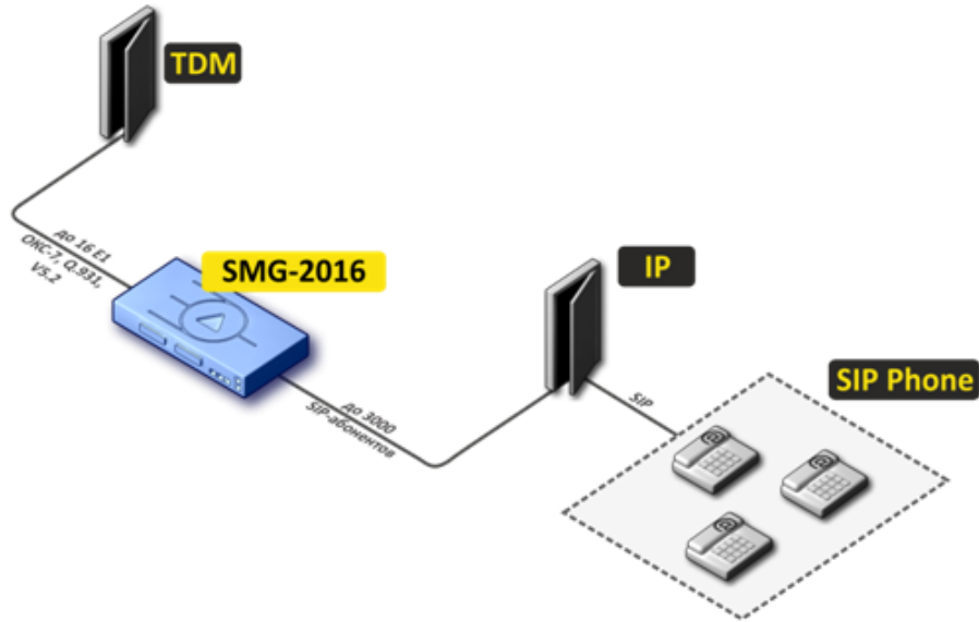
Рисунок 4 – Мини IP-РВХ на базе SMG-2016
