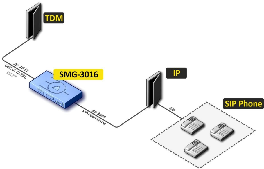
Рисунок 5 – Мини IP-РВХ на базе SMG-3016
