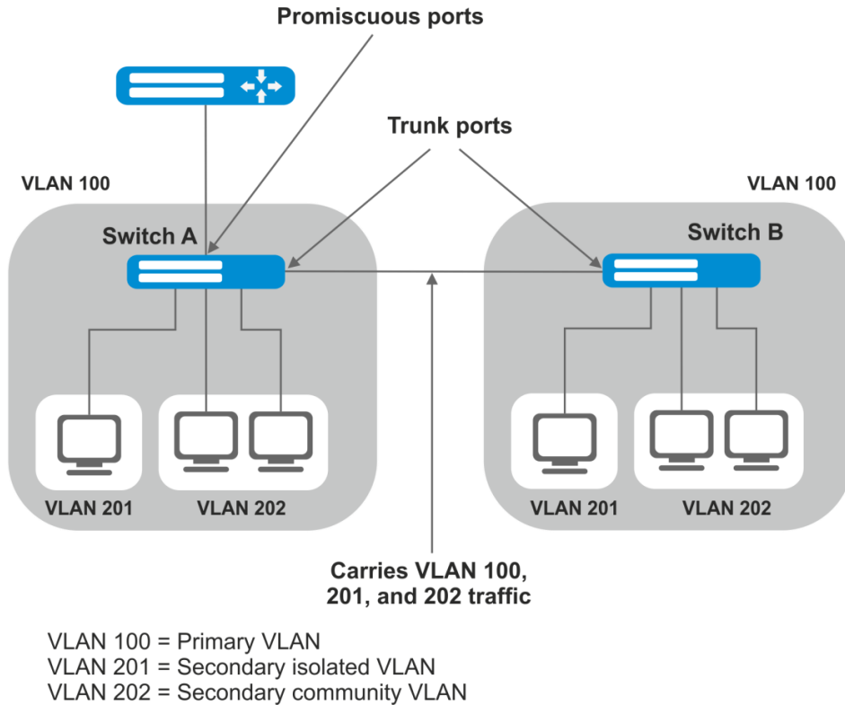
Рисунок 70 – Пример работы технологии Private VLAN
