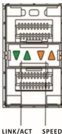
Рисунок 55 – Внешний вид сдвоенного разъема SFP/SFP+/SFP28
