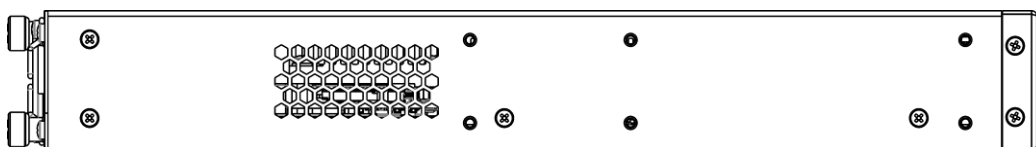
Рисунок 49 – Левая боковая панель MES5400-24
