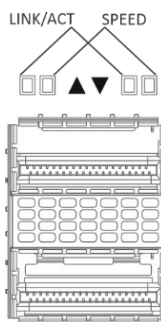
Рисунок 57 – Внешний вид разъема QSFP+ и QSFP28 для MES5400-xx, MES5410-48
