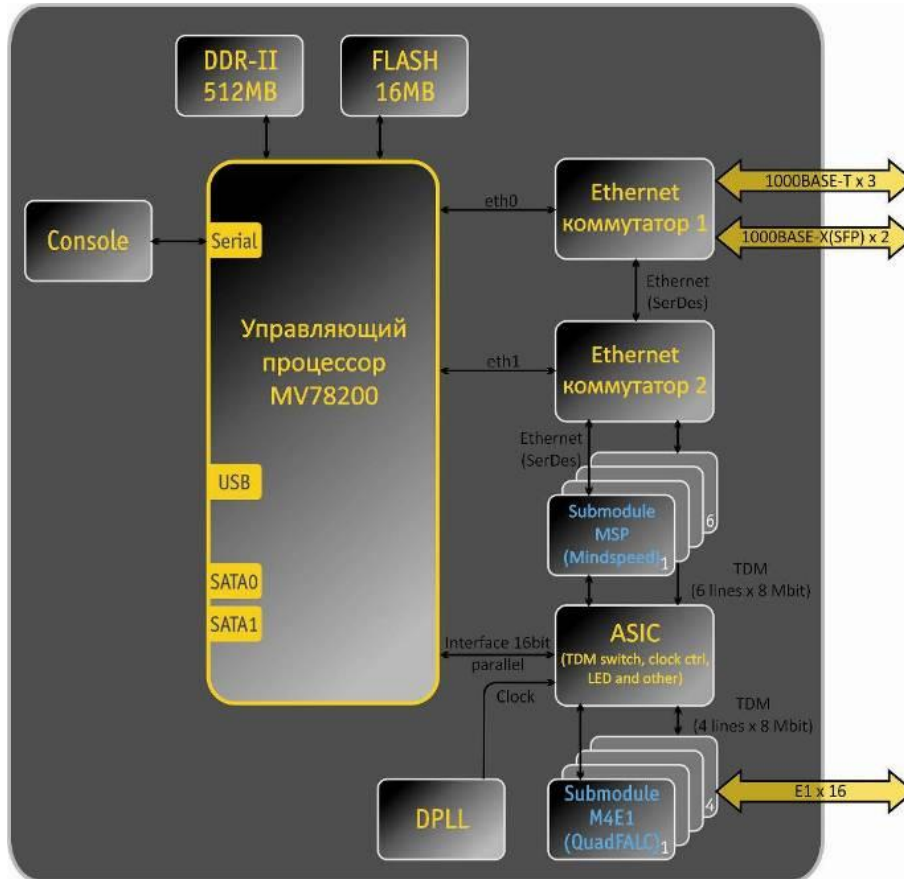
Рисунок 3 – Функциональная схема SMG-1016M-V52AN
