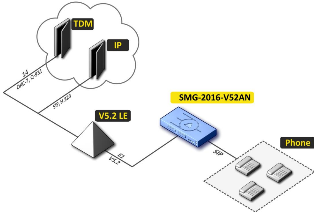
Рисунок 2 – Вынос V5.2 AN на базе SMG-2016-V52AN
