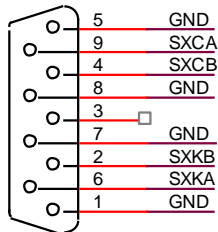
Рисунок 32 – Назначение контактов разъема Console
