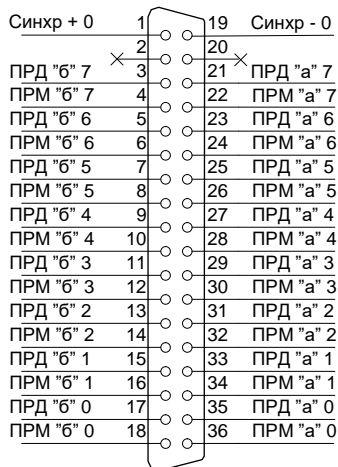
Рисунок 31 – Назначение контактов разъемов E1 Line
