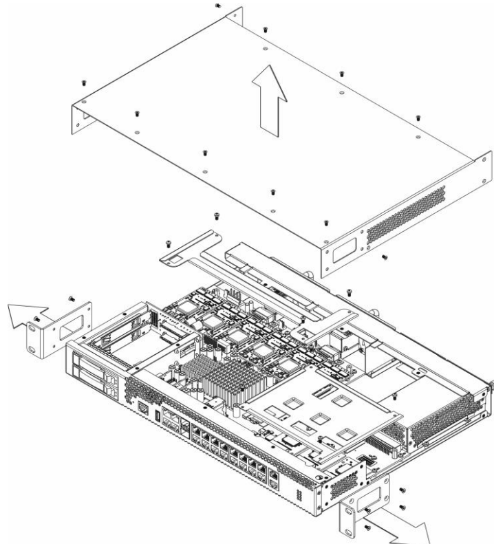
Рисунок 14 – Порядок вскрытия корпуса SMG-2016
