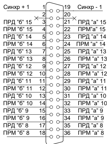
Рисунок 31 – Назначение контактов разъемов E1 Line
