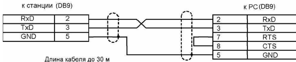
Рисунок 33 – Схема кабеля для подключения к ПОРТ1, ПОРТ2
