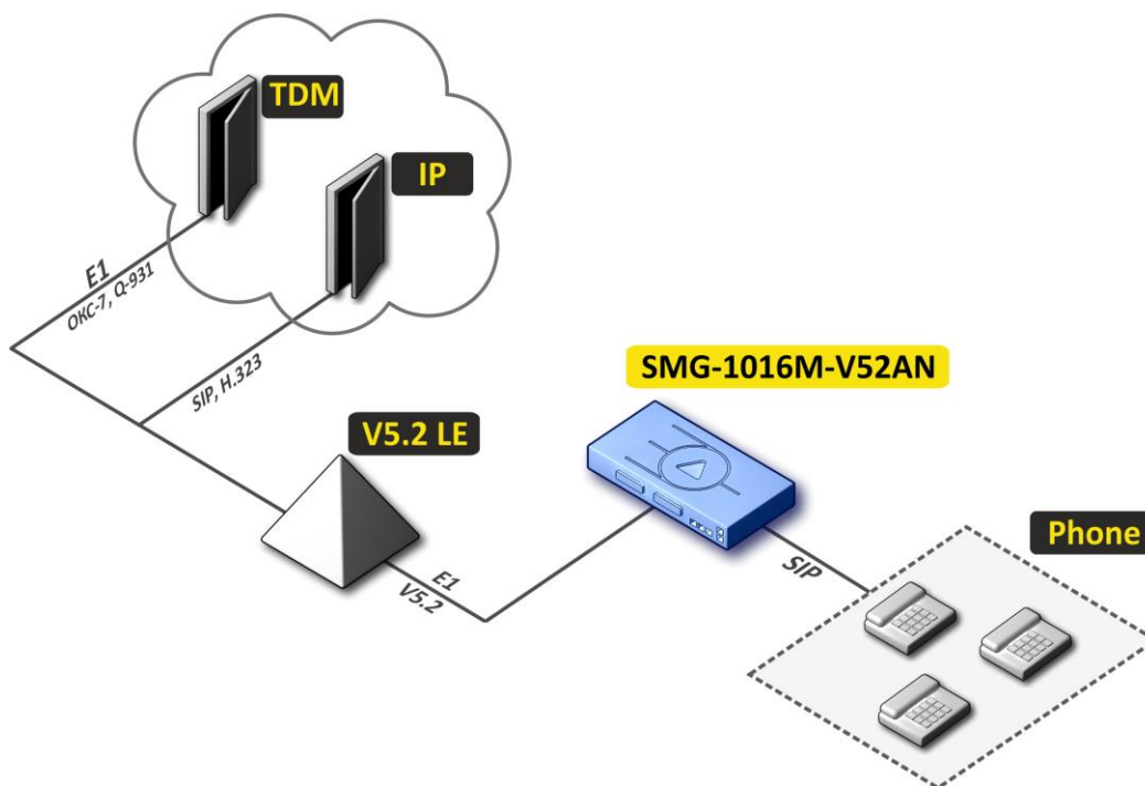
Рисунок 1 – Вынос V5.2 AN на базе SMG-1016M-V52AN
