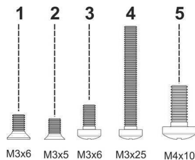
Рисунок 15 – Типы болтов для сборки SMG
