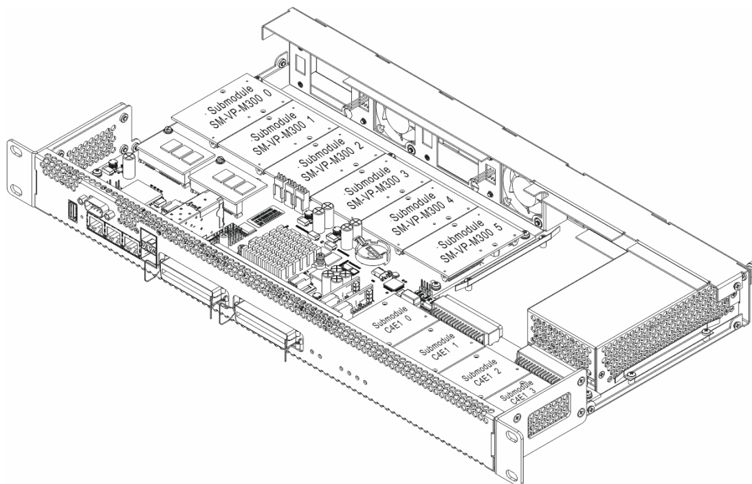
Рисунок 17 – Расположение submodule'ей в SMG-1016M
