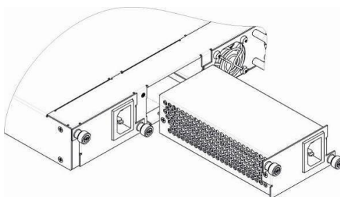
Рисунок 12 – Установка модулей питания
