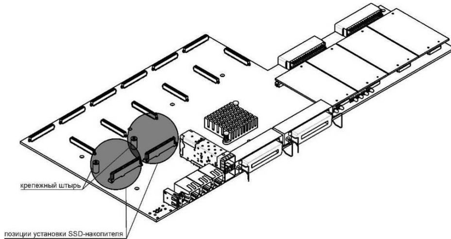
Рисунок 22 – Установка SSD-накопителя
