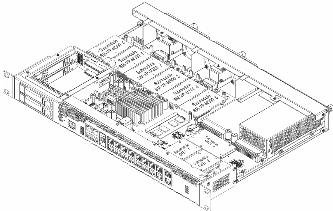
Рисунок 18 – Расположение субмодулей в SMG-2016
