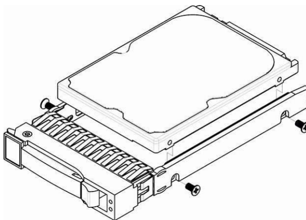
Рисунок 24 – Расположение комплекта крепежных элементов при поставке
