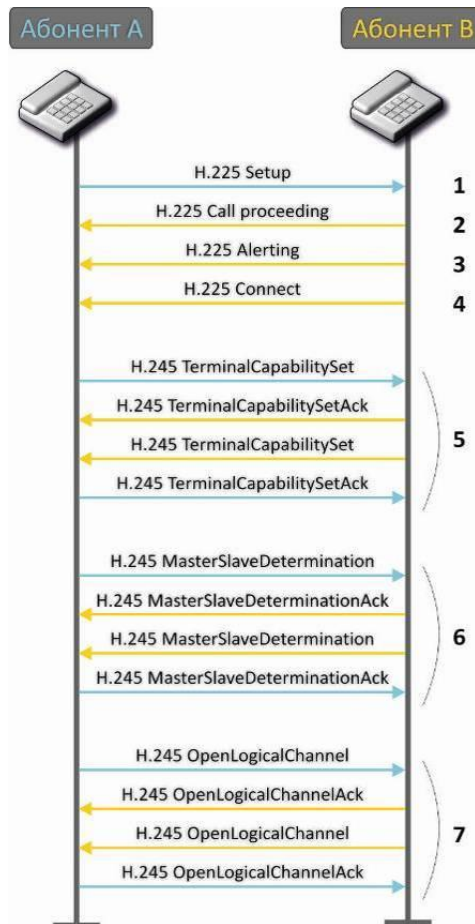
Рисунок 18 – Алгоритм вызова по протоколу H.323
