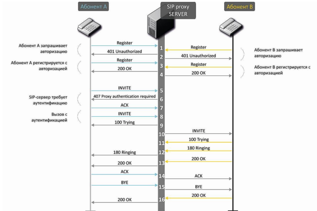
Рисунок 16 – Алгоритм вызова с участием SIP проху-сервера
