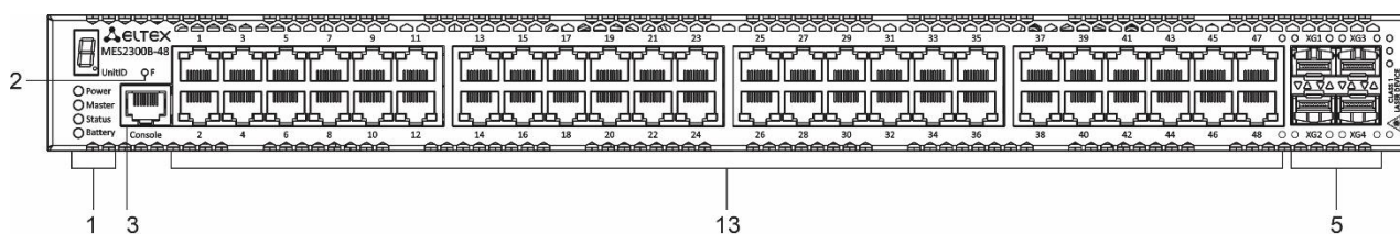
Рисунок 5 – Передняя панель MES2300B-48
