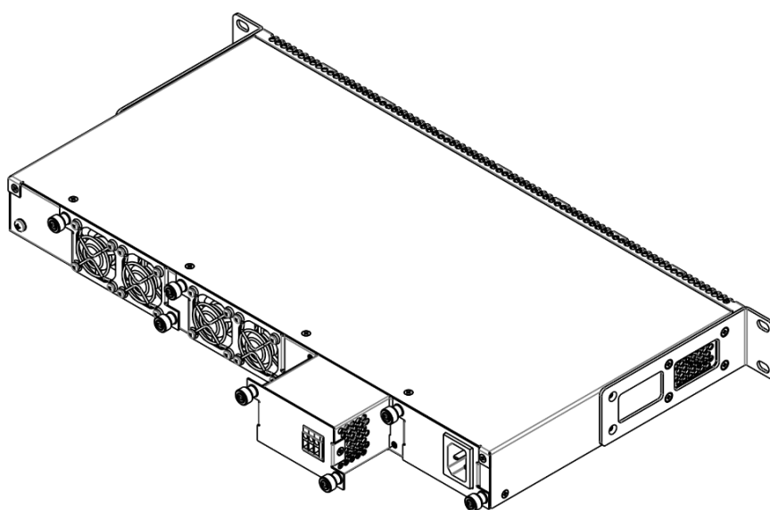
Рисунок 65 – Установка модулей питания
