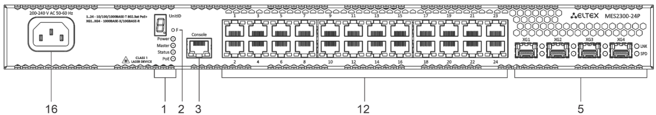
Рисунок 3 – Передняя панель MES2300-24P
