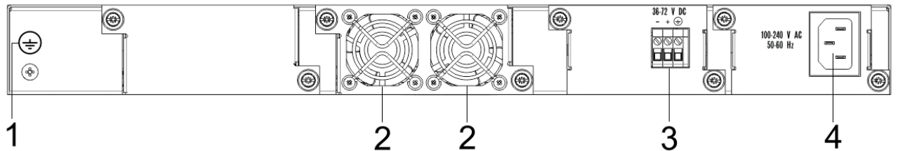
Рисунок 30 – Задняя панель MES5316A
