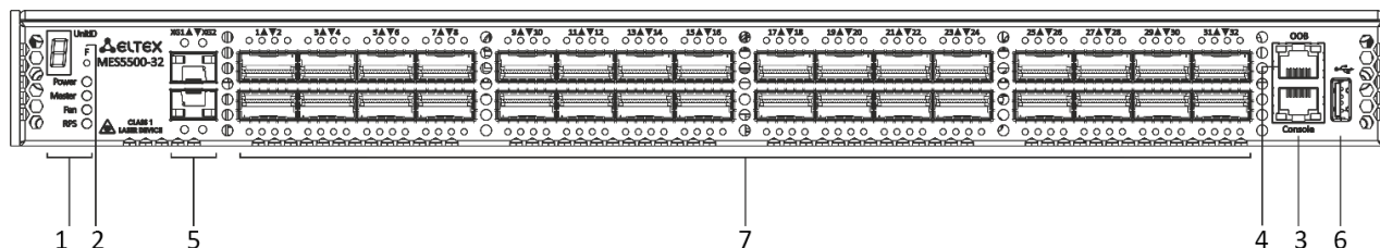
Рисунок 18 – Передняя панель MES5500-32
