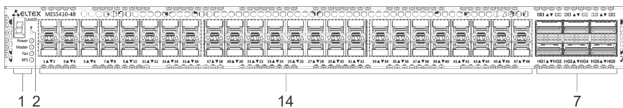
Рисунок 17 – Передняя панель MES5410-48
