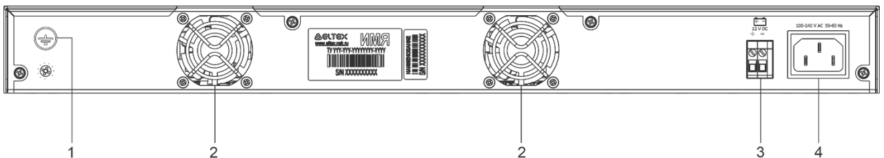
Рисунок 23 – Задняя панель MES2300B-48
