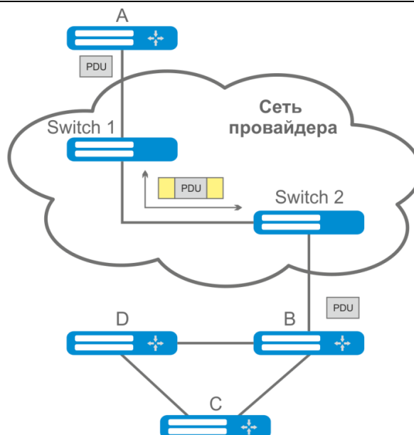
Рисунок 71 — Пример работы функции L2PT
