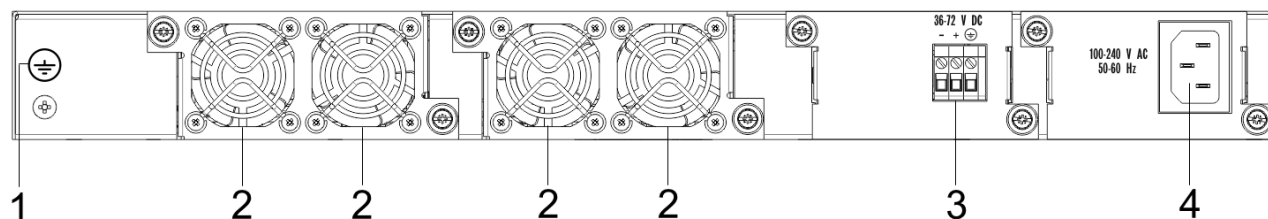
Рисунок 29 – Задняя панель MES5312, MES5324A, MES5332A
