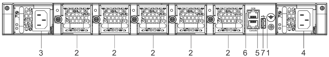
Рисунок 33 – Задняя панель MES5410-48
