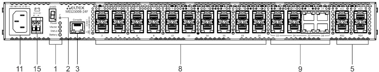
Рисунок 2 – Передняя панель MES2300B-24F
