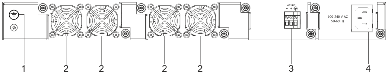
Рисунок 31 – Задняя панель MES5400-24
