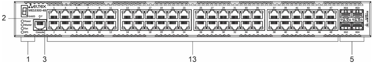
Рисунок 10 – Передняя панель MES3300-48
