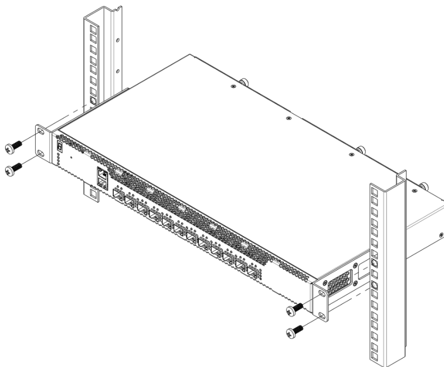
Рисунок 62 – Установка устройства в стойку
