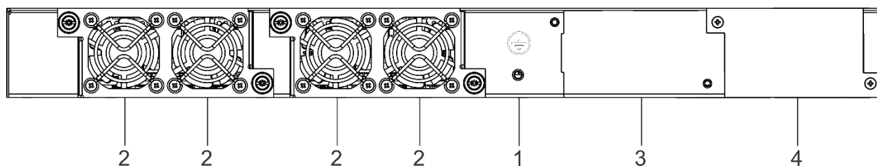
Рисунок 26 – Задняя панель MES3300-16F
