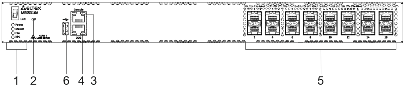
Рисунок 12 – Передняя панель MES5316A
