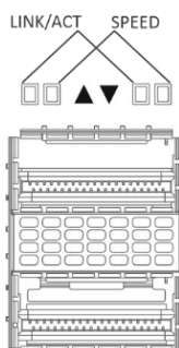
Рисунок 57 – Внешний вид разъема QSFP+ и QSFP28 для MES5400-xx, MES5410-48
