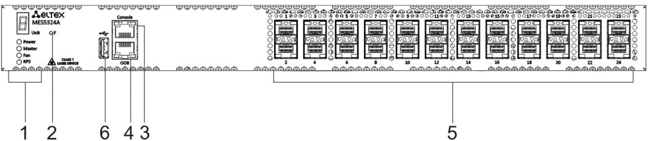
Рисунок 13 – Передняя панель MES5324A
