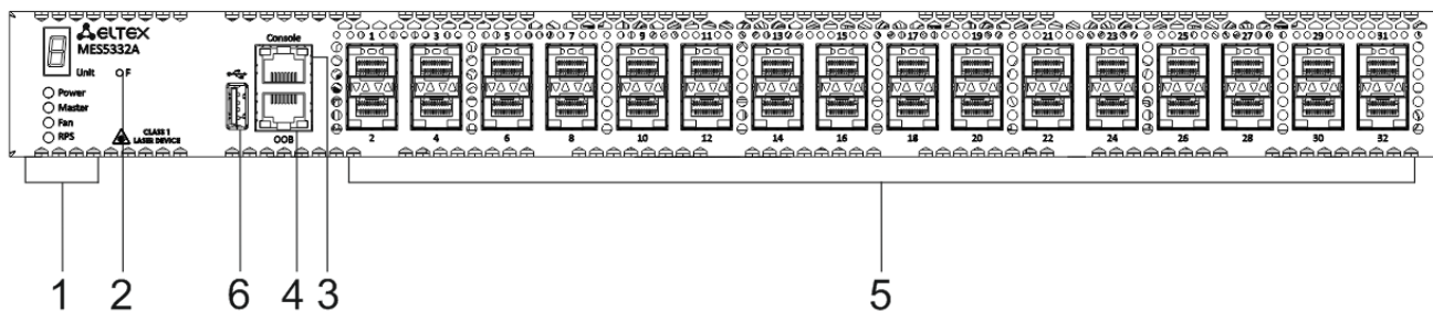
Рисунок 14 – Передняя панель MES5332A
