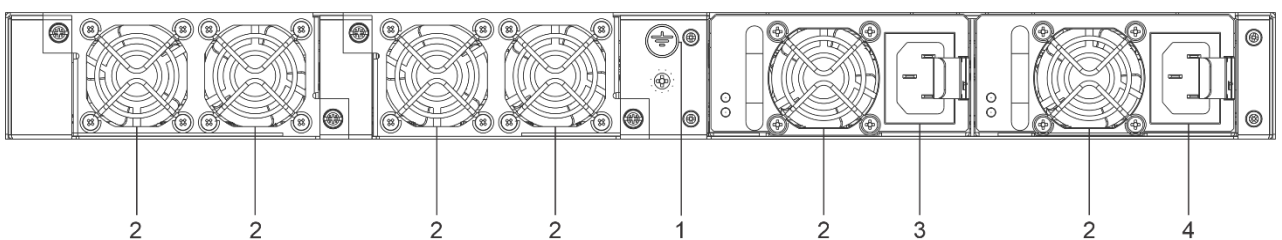
Рисунок 22 – Задняя панель MES2300-48P
