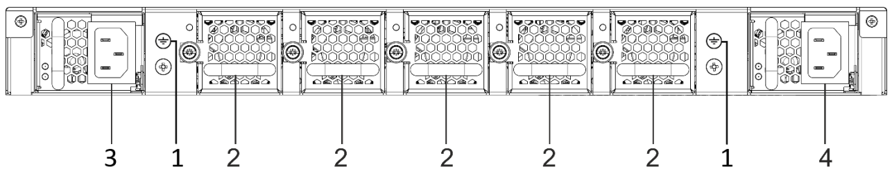
Рисунок 34 – Задняя панель MES5500-32
