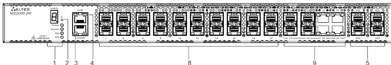
Рисунок 9 – Передняя панель MES3300-24F
