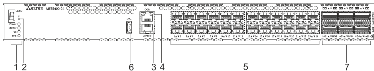
Рисунок 15 – Передняя панель MES5400-24
