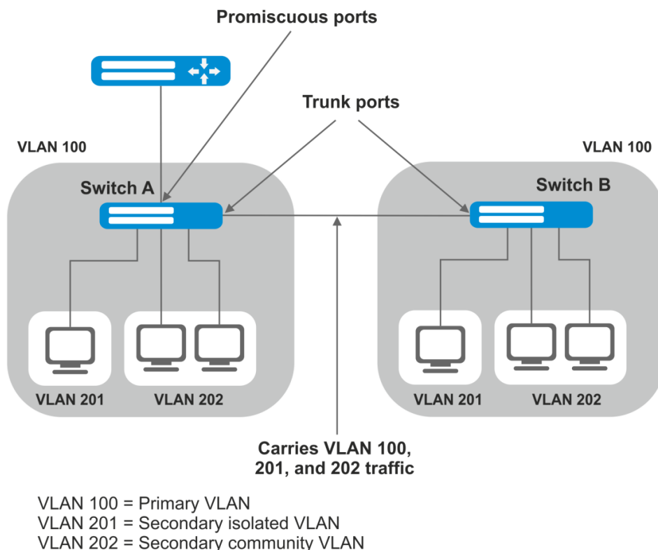
Рисунок 70 – Пример работы технологии Private VLAN
