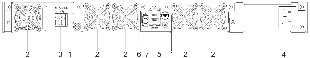
Рисунок 32 – Задняя панель MES5400-48
