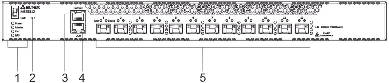
Рисунок 11 – Передняя панель MES5312
