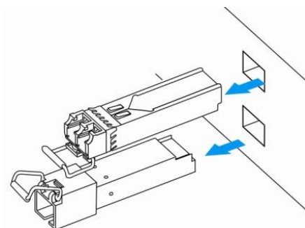
Рисунок 69 – Извлечение SFP-трансиверов
