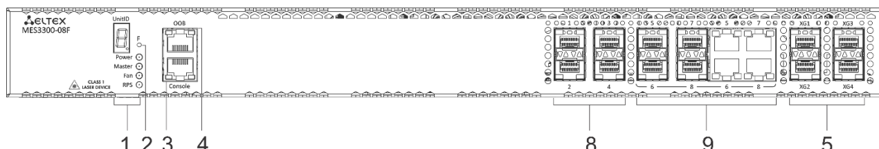
Рисунок 7 – Передняя панель MES3300-08F
