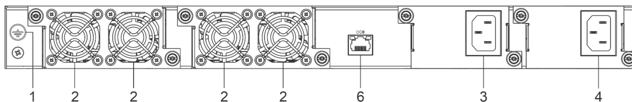
Рисунок 28 – Задняя панель MES3300-48
